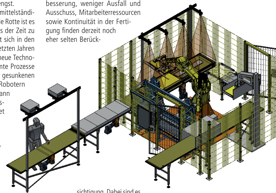
>Roboterzelle mit einer Presse für Schubkästen und Auszüge der Längen 300 bis 1.200 Millimeter und 300er, 400er und 500er Tiefe mit Bediener-Assistenzsystem für die Teilaufgabe. Die Beschickung erfolgt „just in sequence“ nach Vorgabe durch ein Leitrechnersystem.
